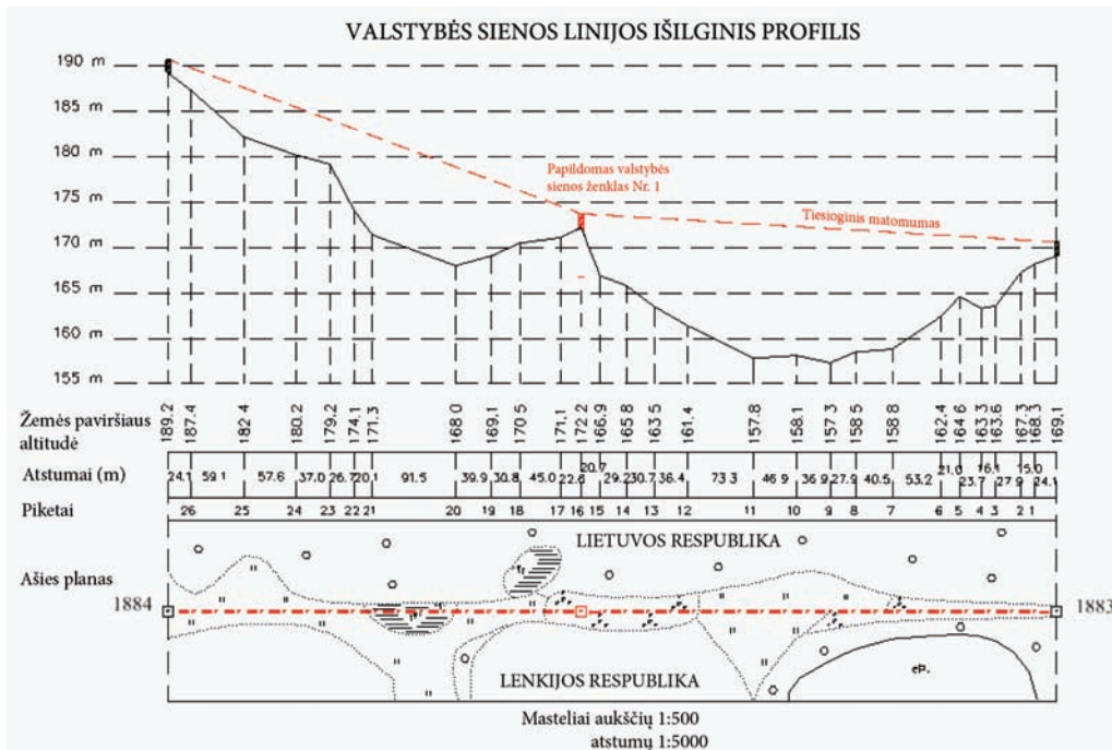
6 pav. Sienos linijos išilginis profilis
